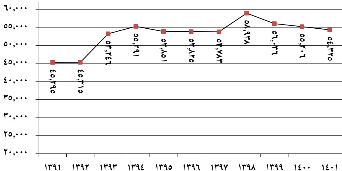
نمودار روند تولید M.D.F (مترمکعب) طی سالهای ۱۳۹۱ الی ۱۴۰۱
