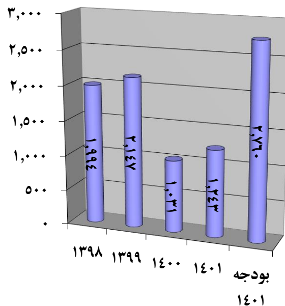
نمودار مقایسه مقدار تولید ورق فوم برد (تن) با بودجه سال ۱۴۰۱
